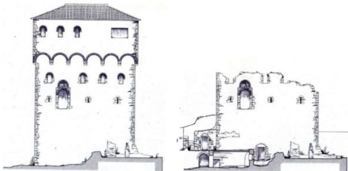
Εικ 23: Αναπαράσταση μορφής πύργου βάσει σχεδίου Barsky. Χ. Μπούρας – Η Νέα Μονή της Χίου, Ιστορία και Αρχιτεκτονική (1981)
