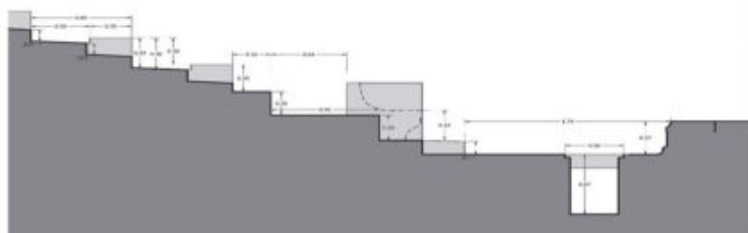
8.Σχεδιαστική τομή του θεάτρου
