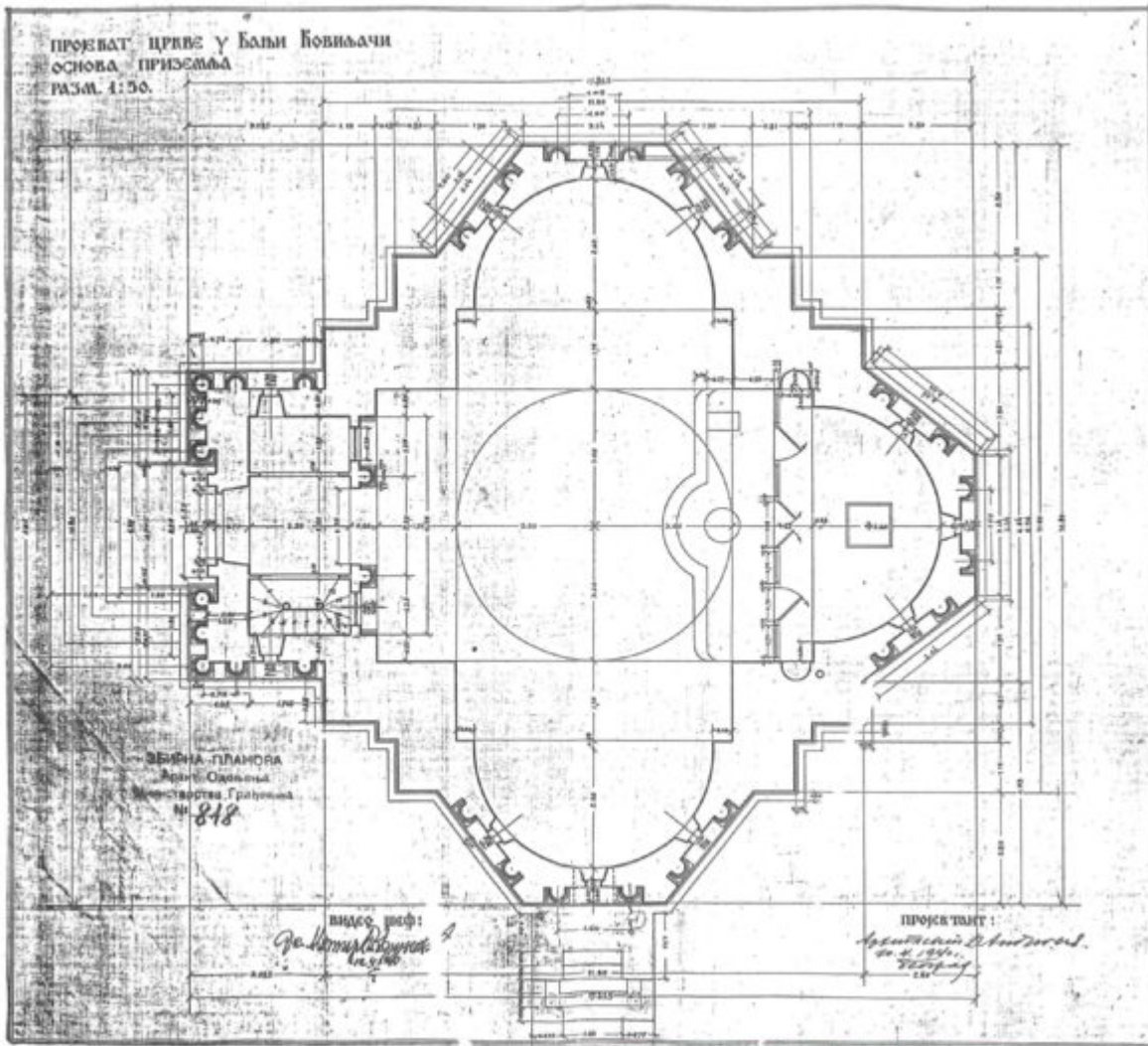
Пројекат старог храма Светог Ђорђа у Бањи Ковиљачи
