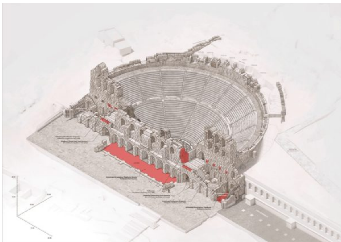
Προτεινόμενες καθαιρέσεις προγενέστερων επεμβάσεων στο μνημείο
