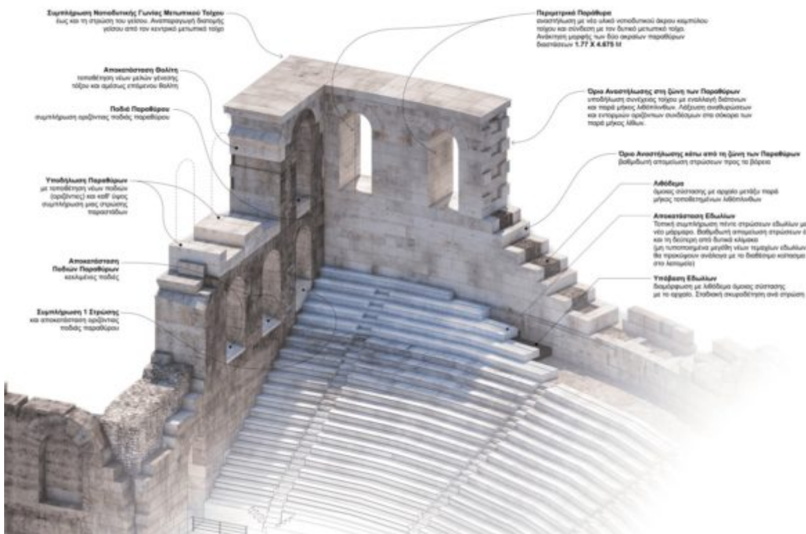
Πρόταση αναστήλωσης νοτιοδυτικής γωνίας Κούλου
