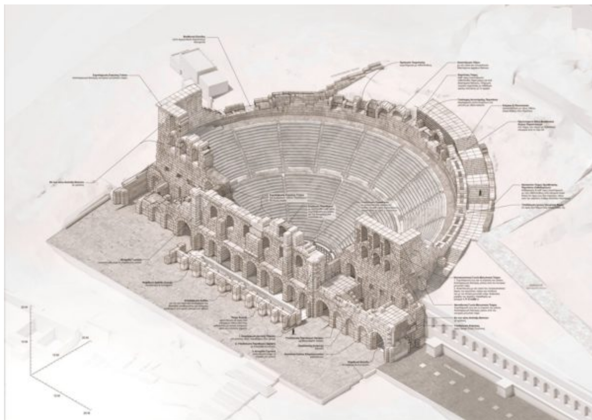
Πρόταση αναστήλωσης
