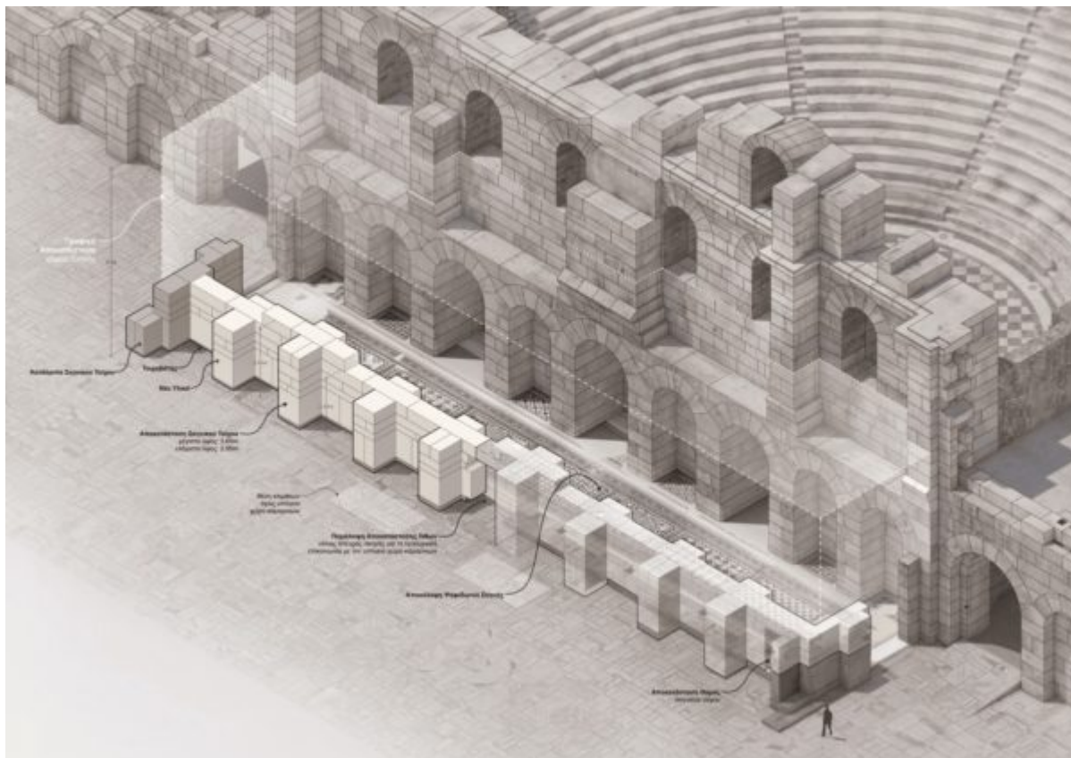
Πρόταση αναστήλωσης Σκηηνής
