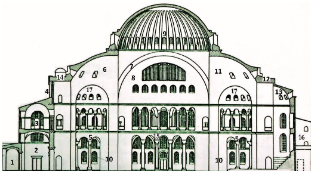
Σχῆμα Η. Ἐπιμήκης τομή τοῦ ναοῦ.
