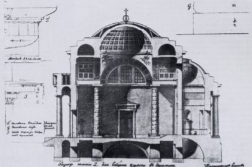
Чертеж сечения I. для Св. Спаса и Св. Духа
