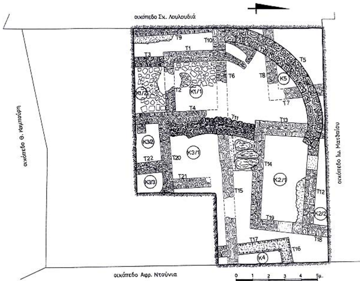
Τένεδος. Κάτοψη της ανασκαφής στο οικόπεδο Π. Λουλουδιά. Δεκέμβριος 2001
